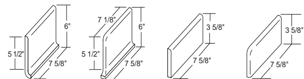
Q3585 Cove Base Q3585 L/R Cove Base Outside Corner Q1485 Bullnose Q1485 L/R Bullnose Corner
